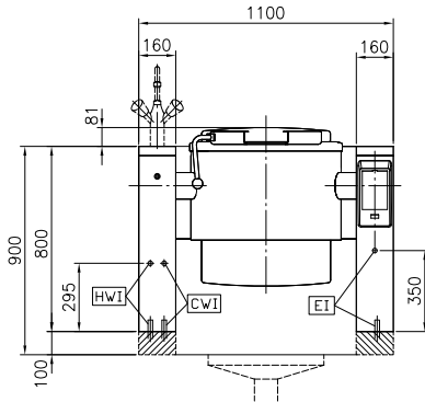
Front aanzicht
