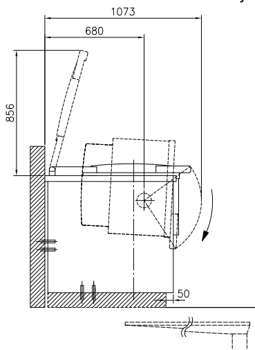
Zij aanzicht
